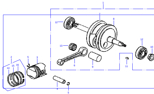
F10 Crankshaft & Piston
